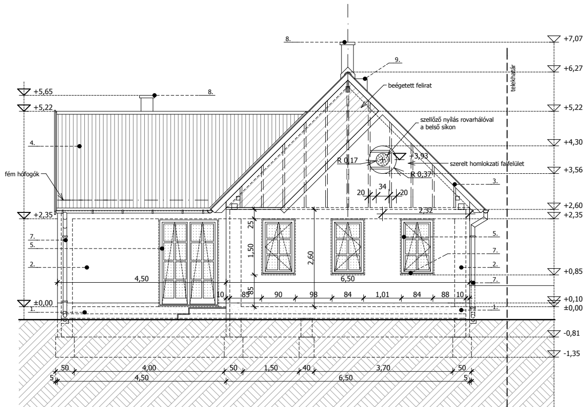
KELETI HOMLOKZAT
