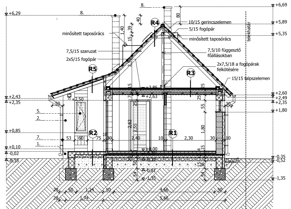
A - A METSZET
