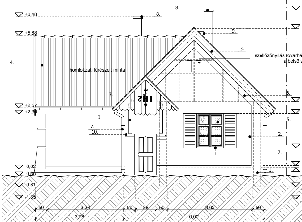
UTCA FELŐLI HOMLOKZAT
