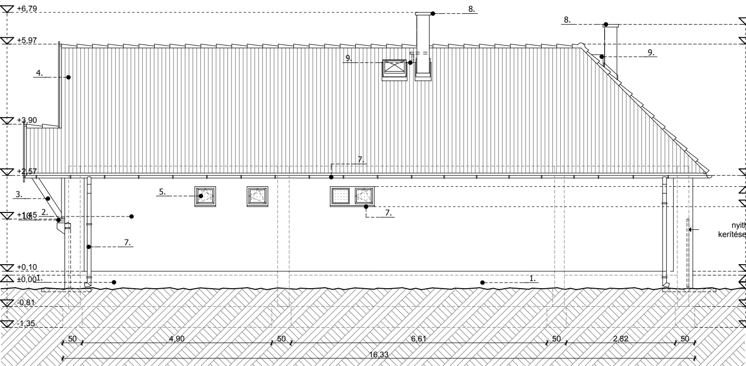
OLDALSÓ HOMLOKZAT
