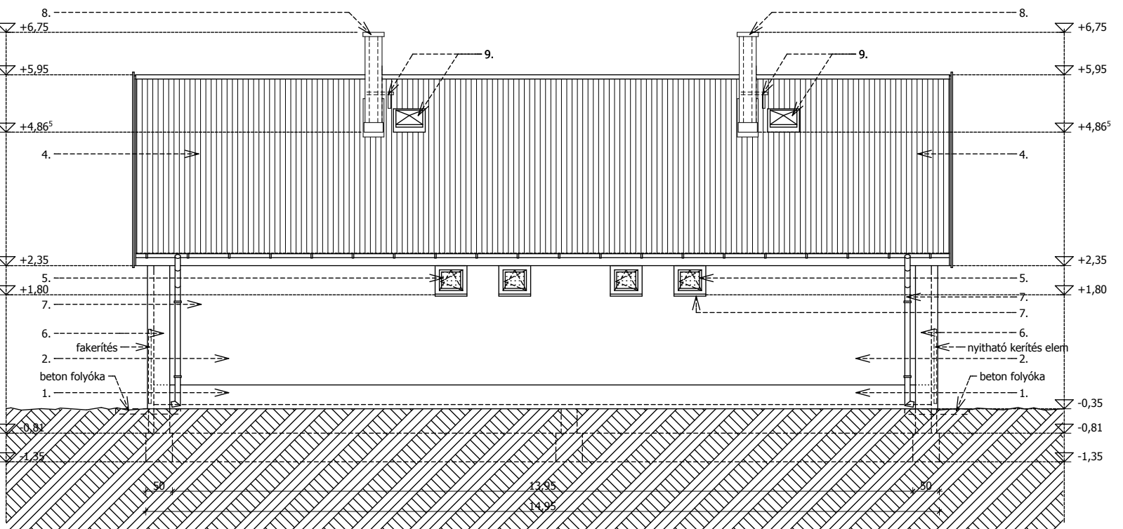
OLDAL HOMLOKZAT
