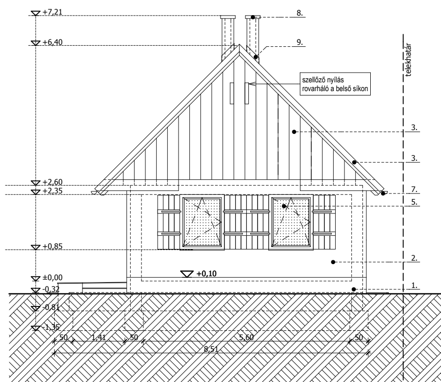
KELETI HOMLOKZAT
