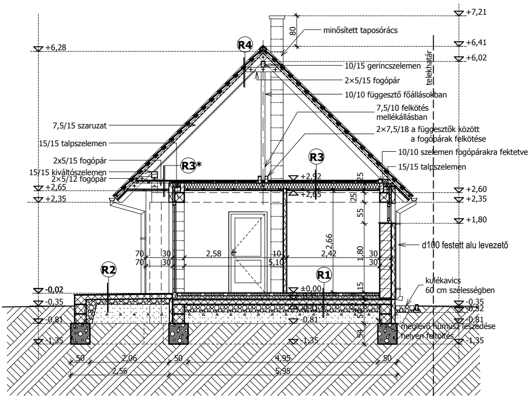
A - A METSZET
