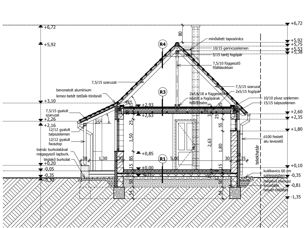
A - A KERESZTMETSZET
