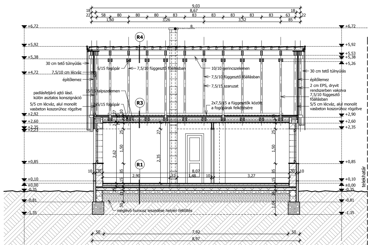
B - B HOSSZMETSZET
