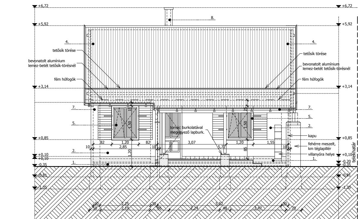
DÉLI HOMLOKZAT
