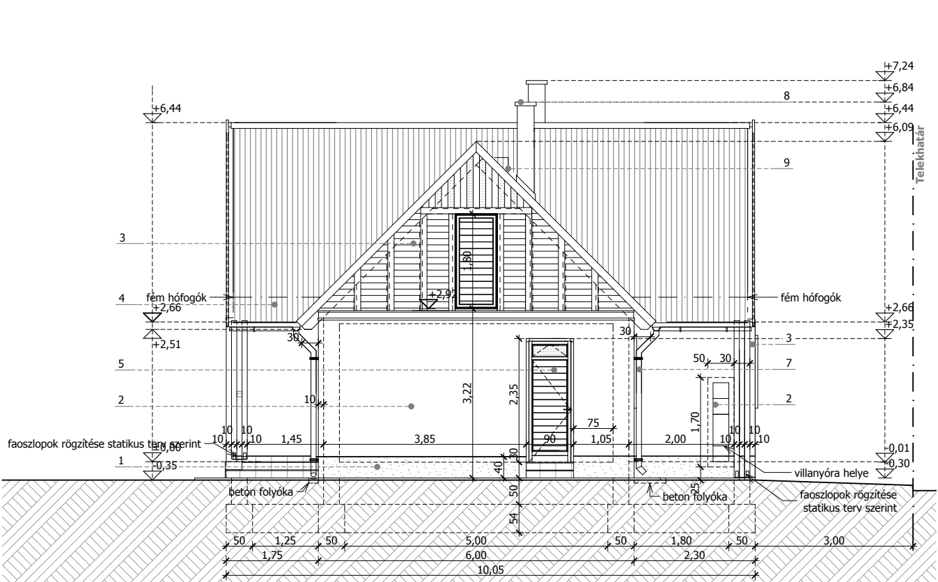
DÉLI HOMLOKZAT
