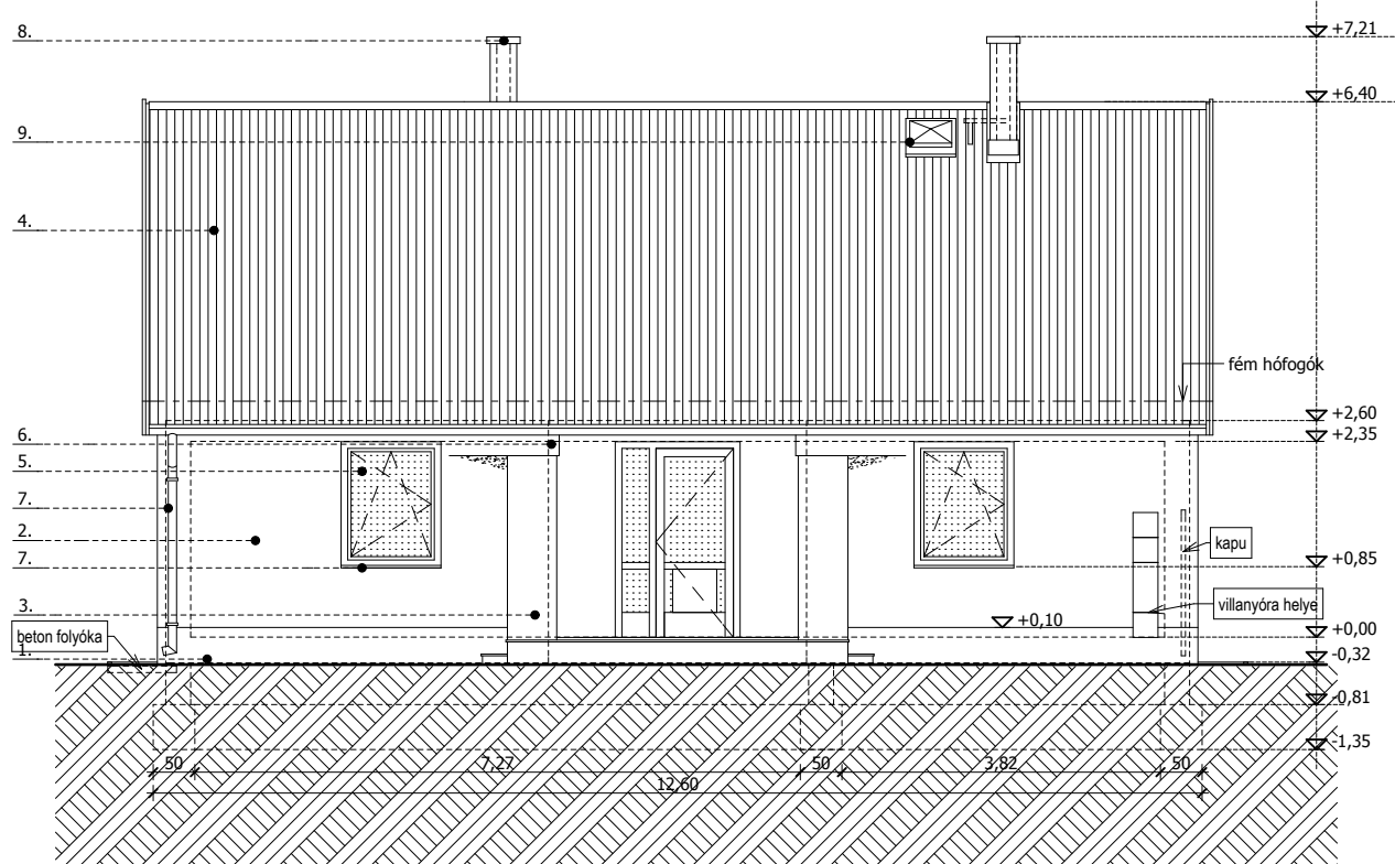
DÉLI HOMLOKZAT
