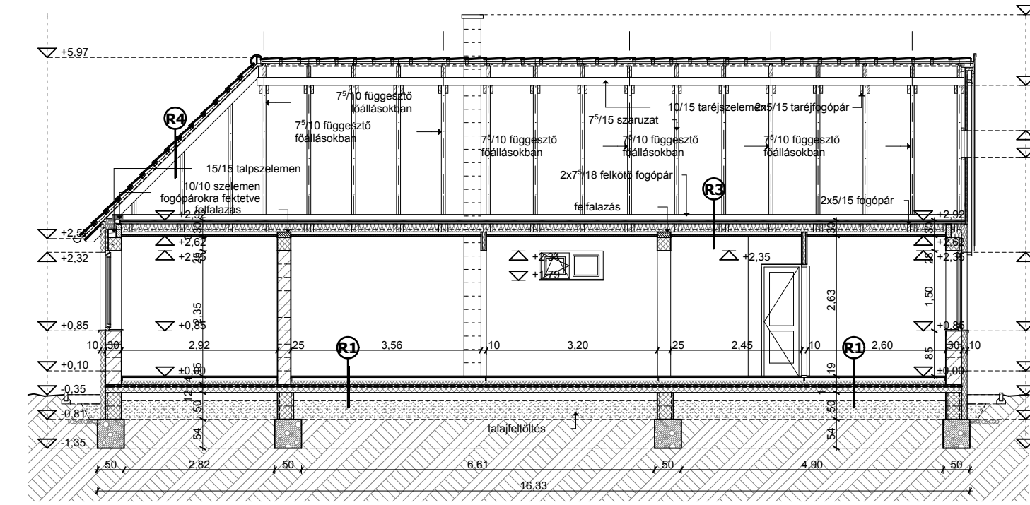
B - B METSZET
