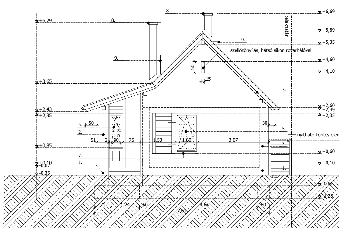
KELETI HOMLOKZAT
