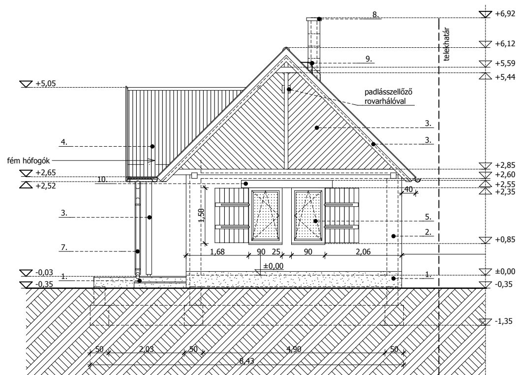
KELETI HOMLOKZAT
