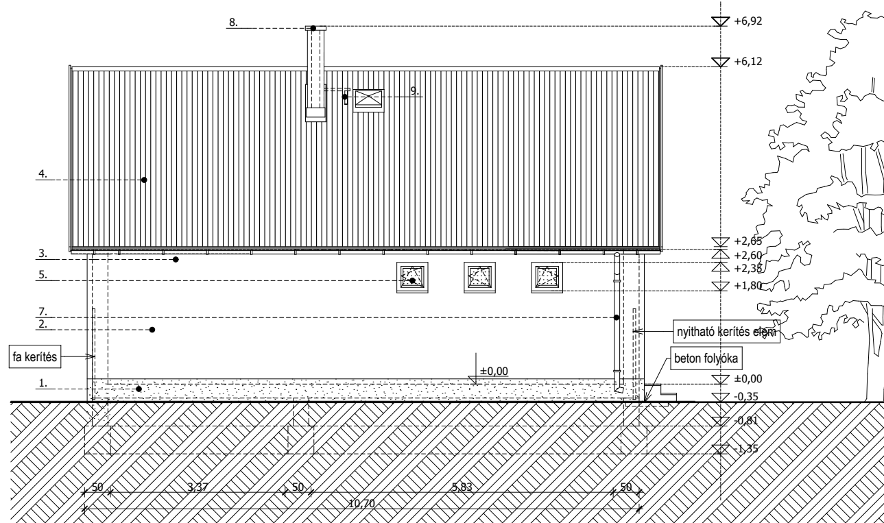
ÉSZAKI HOMLOKZAT
