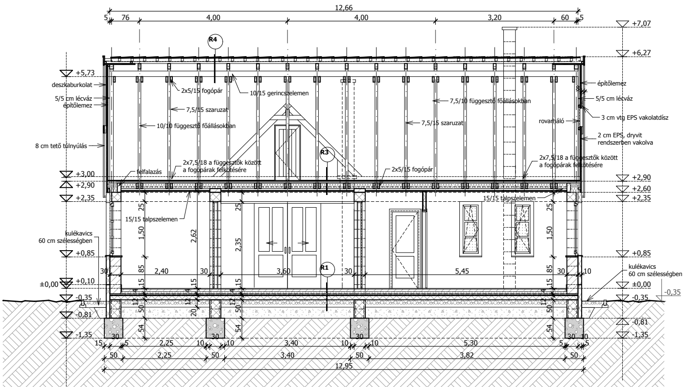
B-B HOSSZMETSZET
