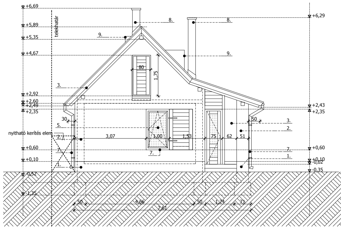
NYUGATI HOMLOKZAT
