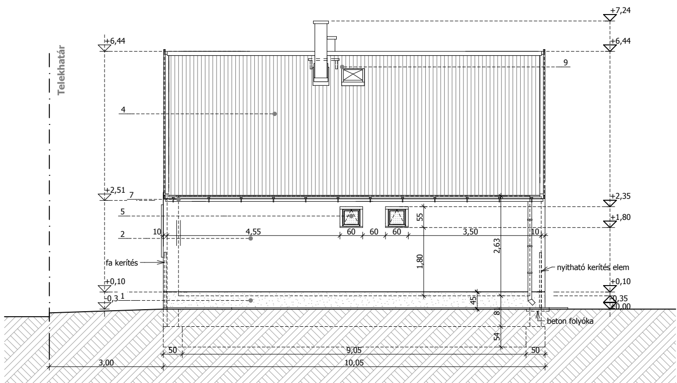
ÉSZAKI HOMLOKZAT
