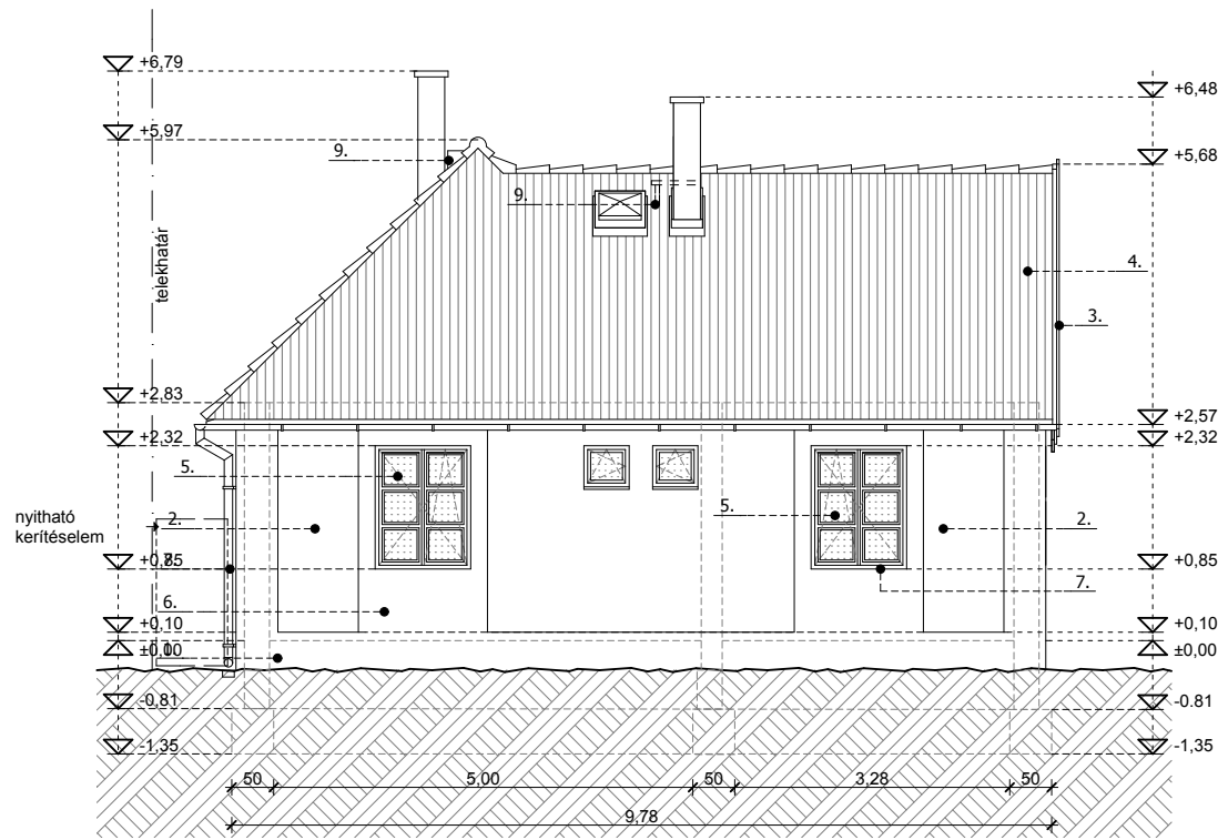
HÁTSÓ HOMLOKZAT
