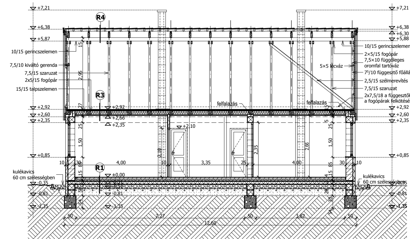
B - B HOSSZMETSZET
