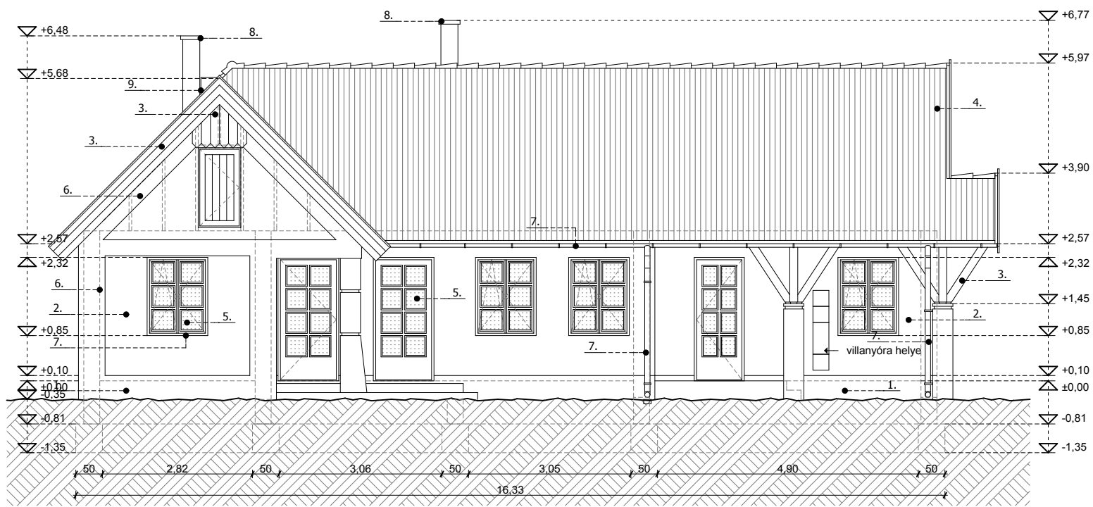
UDVARI HOMLOKZAT
