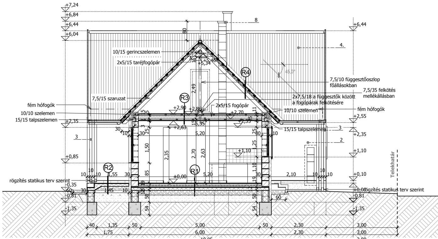
A - A METSZET
