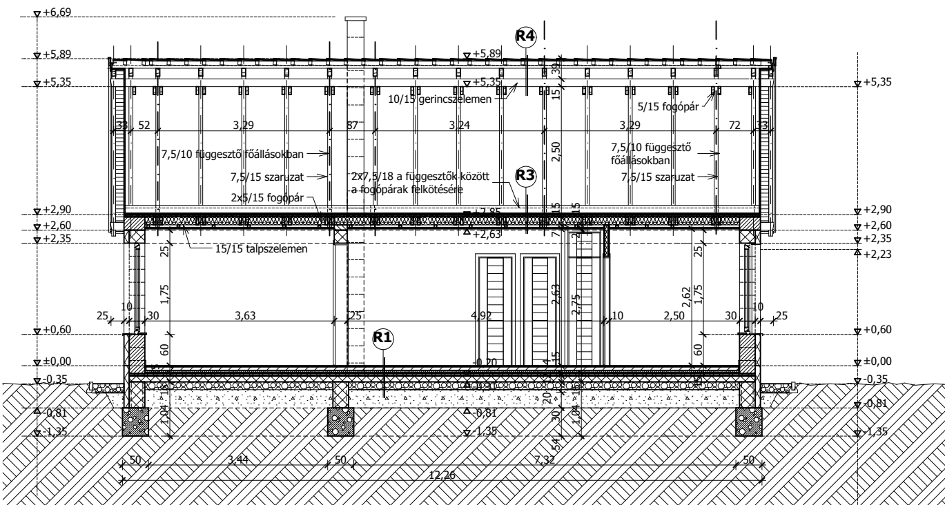
B - B HOSSZMETSZET
