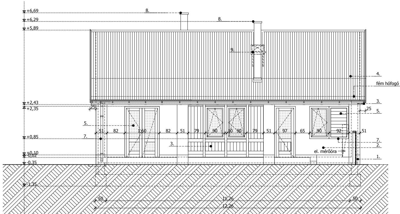
DÉLI HOMLOKZAT
