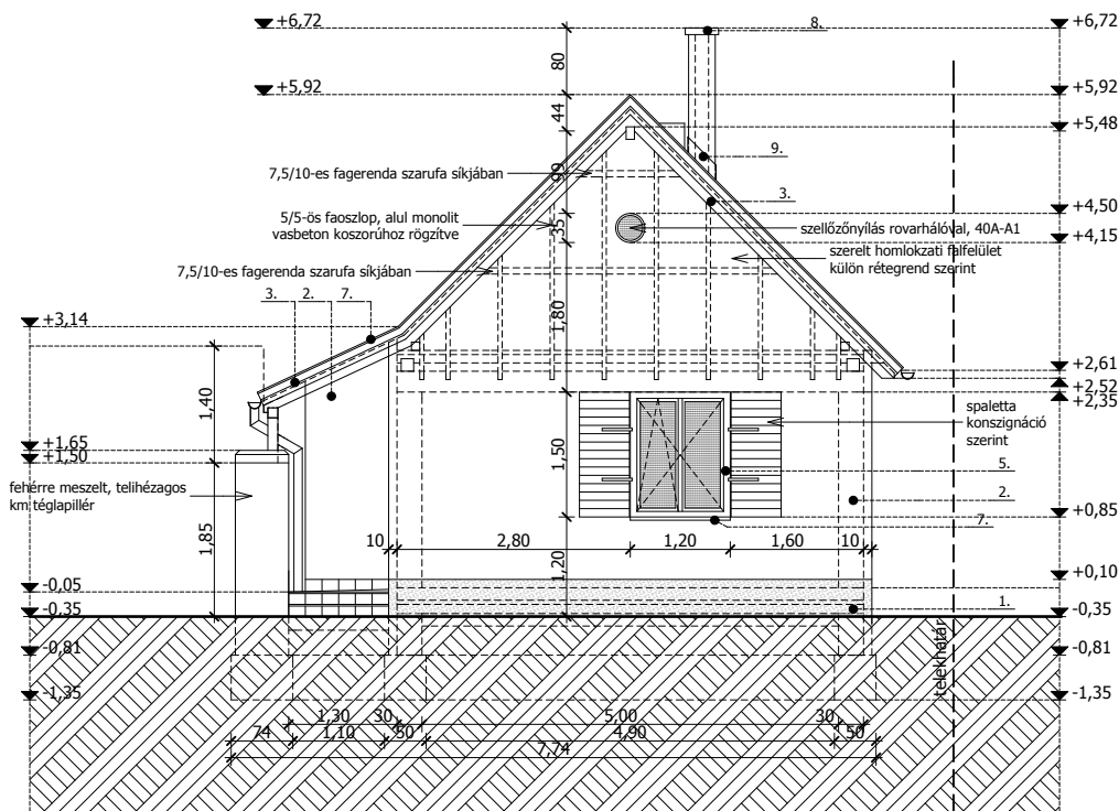
KELETI HOMLOKZAT
