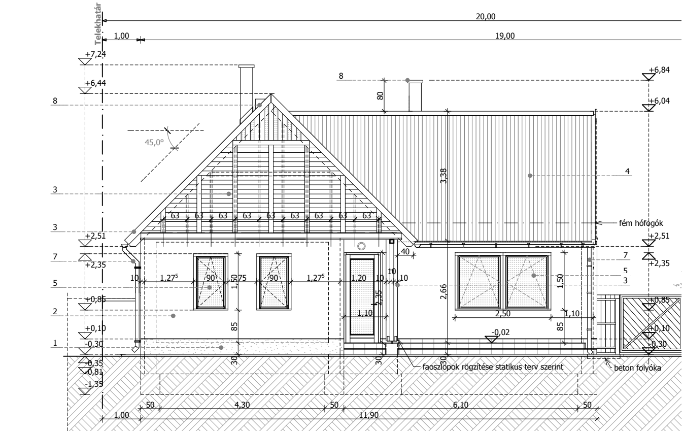
NYUGATI HOMLOKZAT
