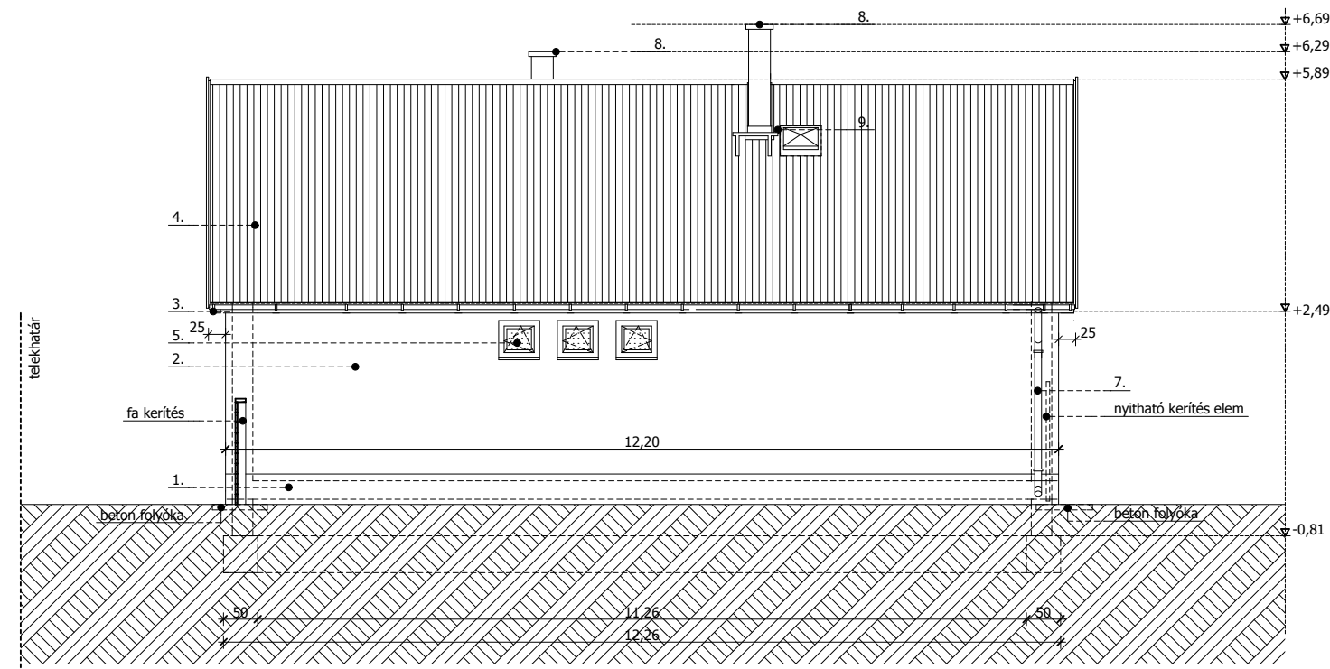
ÉSZAKI HOMLOKZAT
