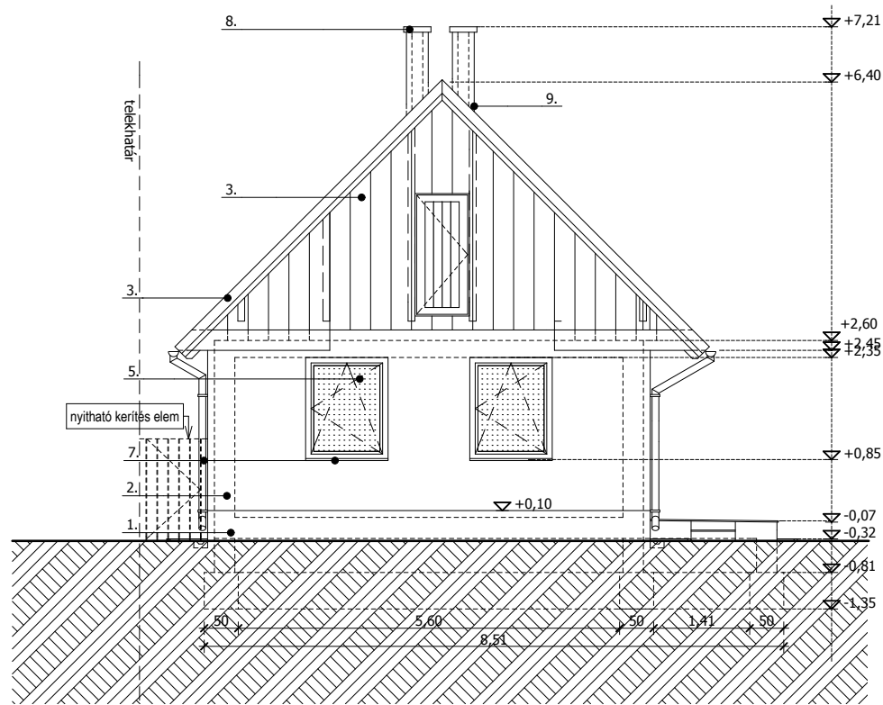
NYUGATI HOMLOKZAT
