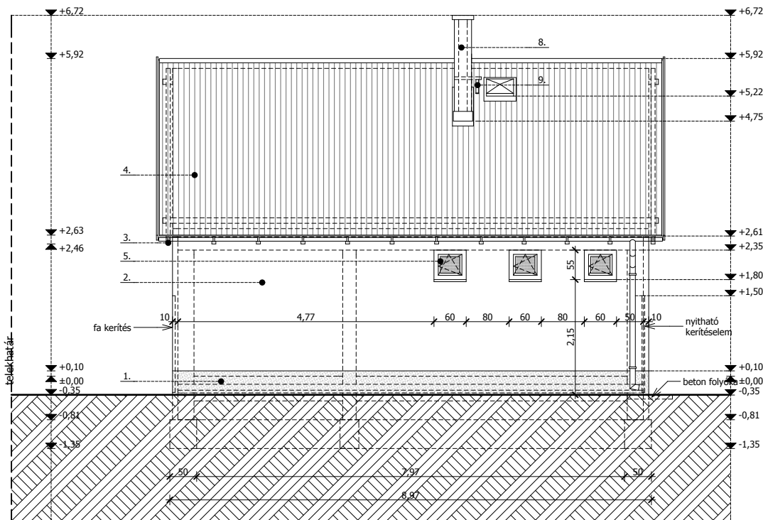
ÉSZAKI HOMLOKZAT
