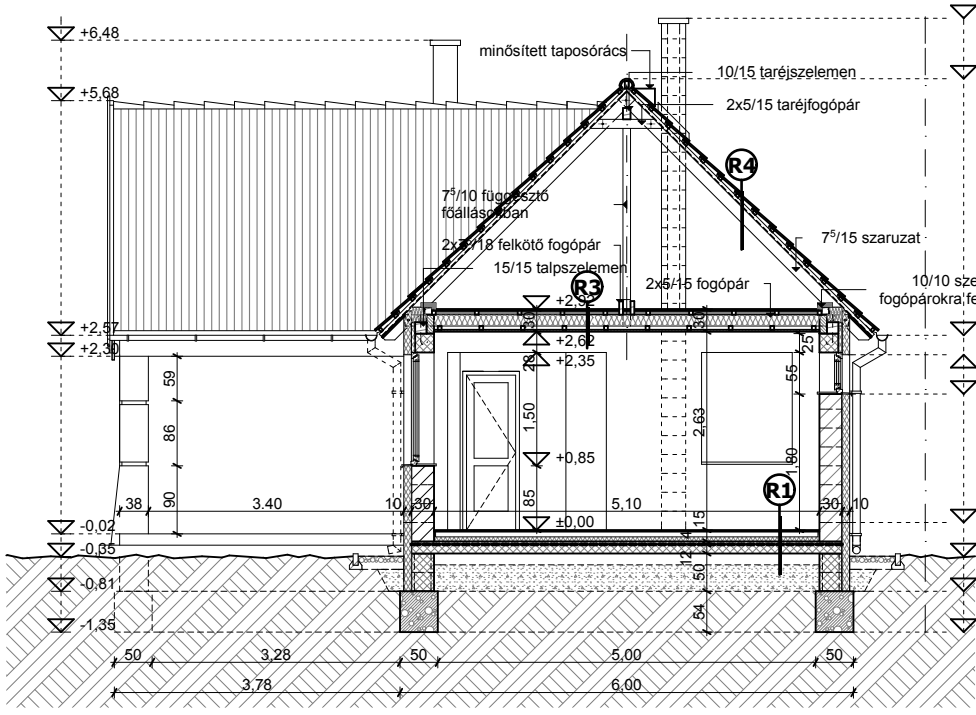
A - A METSZET
