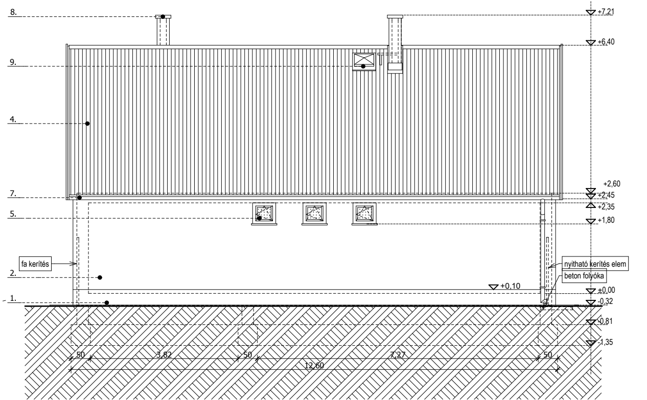
ÉSZAKI HOMLOKZAT
