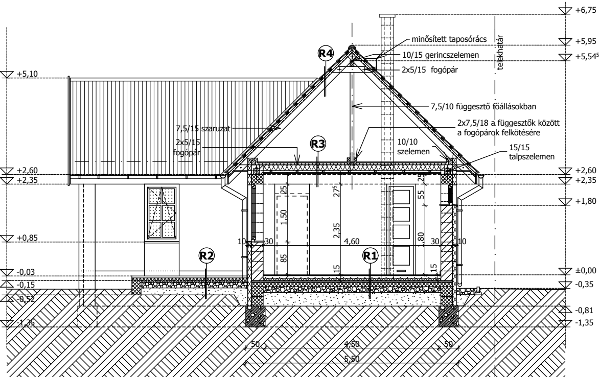
A-A METSZET
