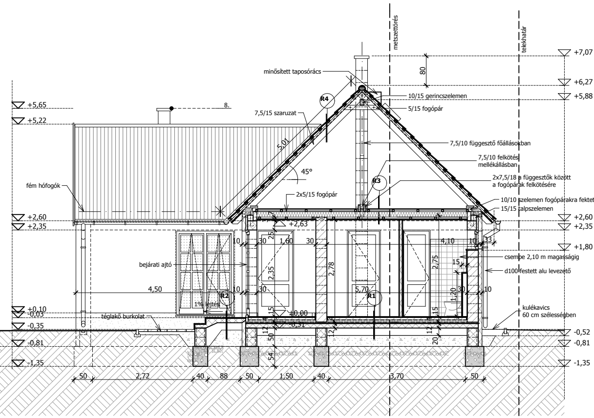
A-A METSZET
