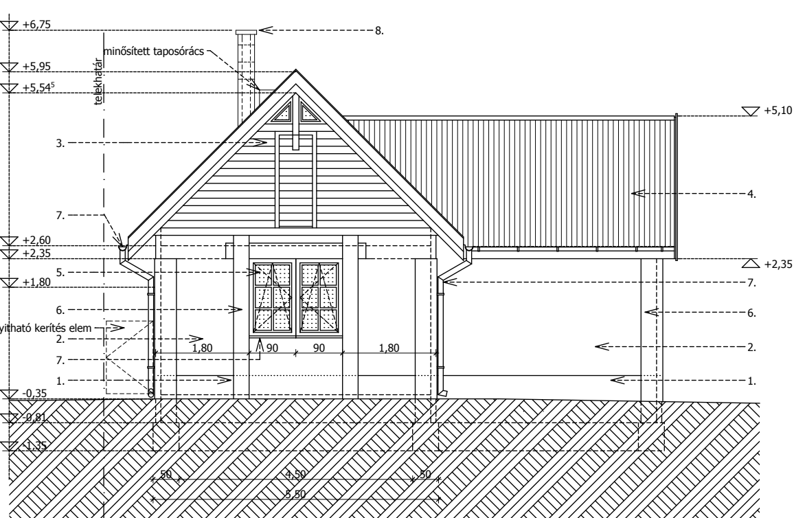
HÁTSÓ HOMLOKZAT
