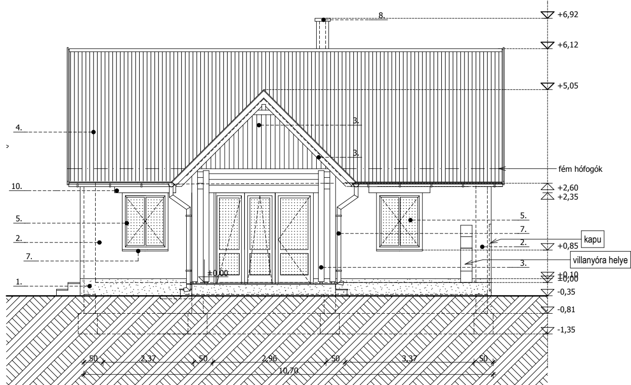
DÉLI HOMLOKZAT
