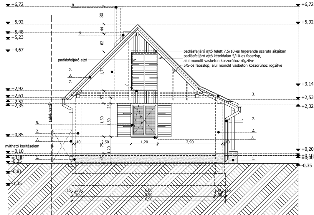
NYUGATI HOMLOKZAT
