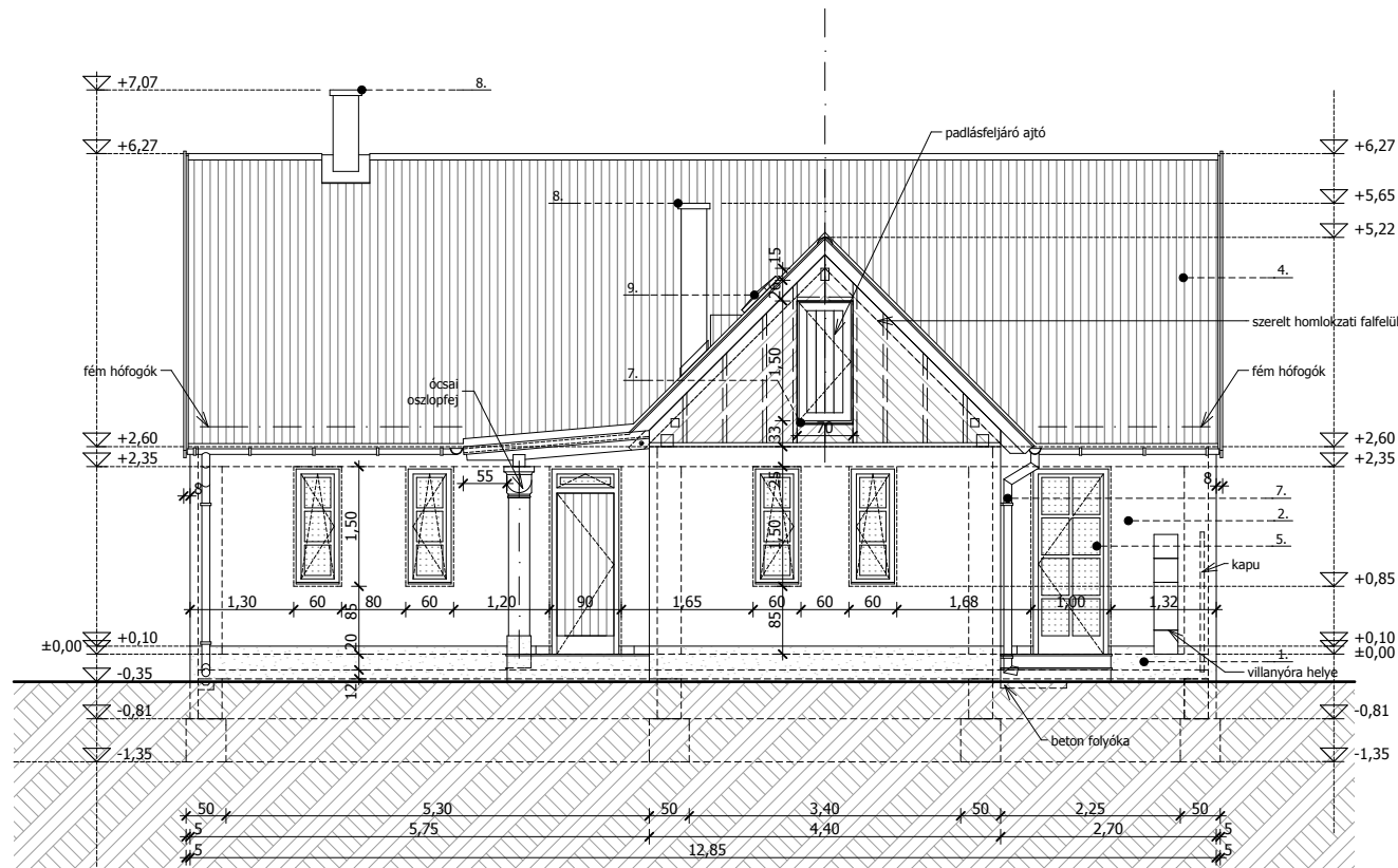
DÉLI HOMLOKZAT
