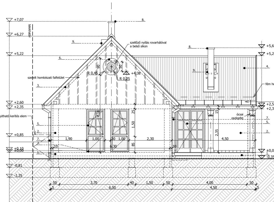
NYUGATI HOMLOKZAT
