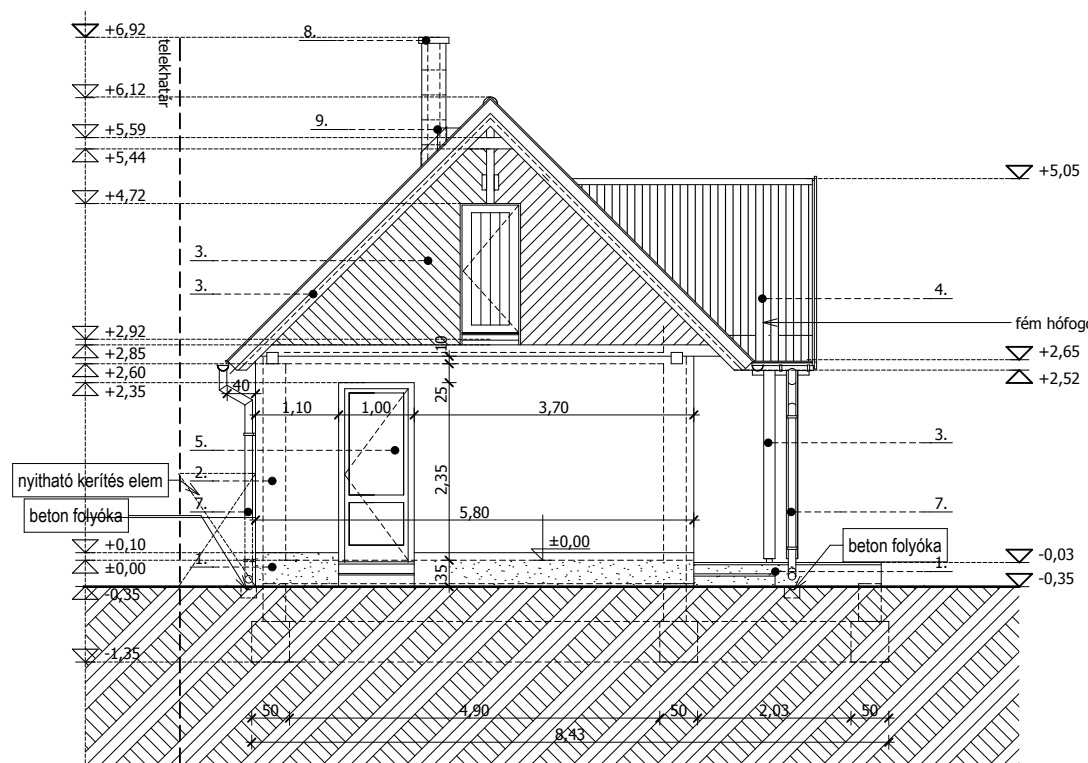
NYUGATI HOMLOKZAT
