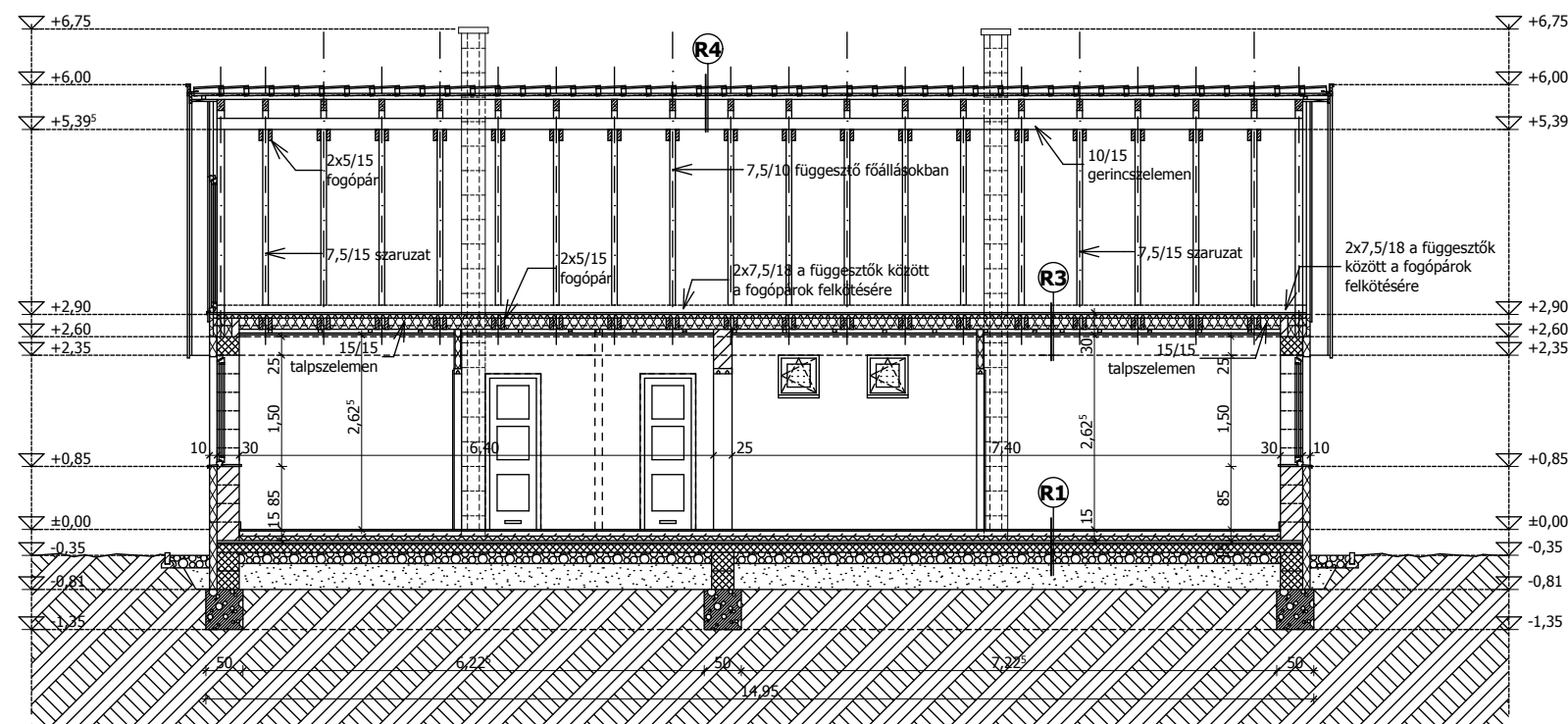
B-B HOSSZMETSZET
