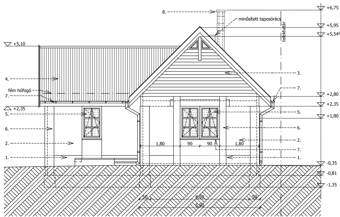
UTCAI HOMLOKZAT
