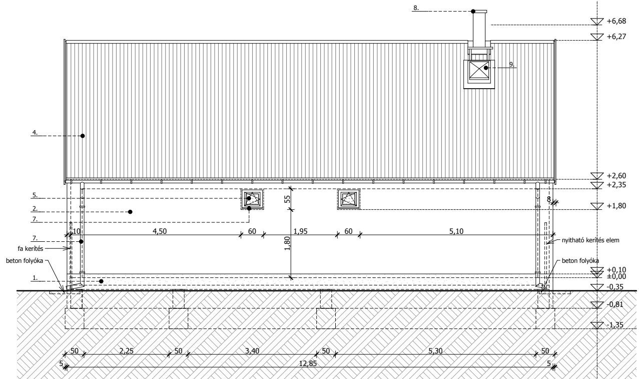
ÉSZAKI HOMLOKZAT
