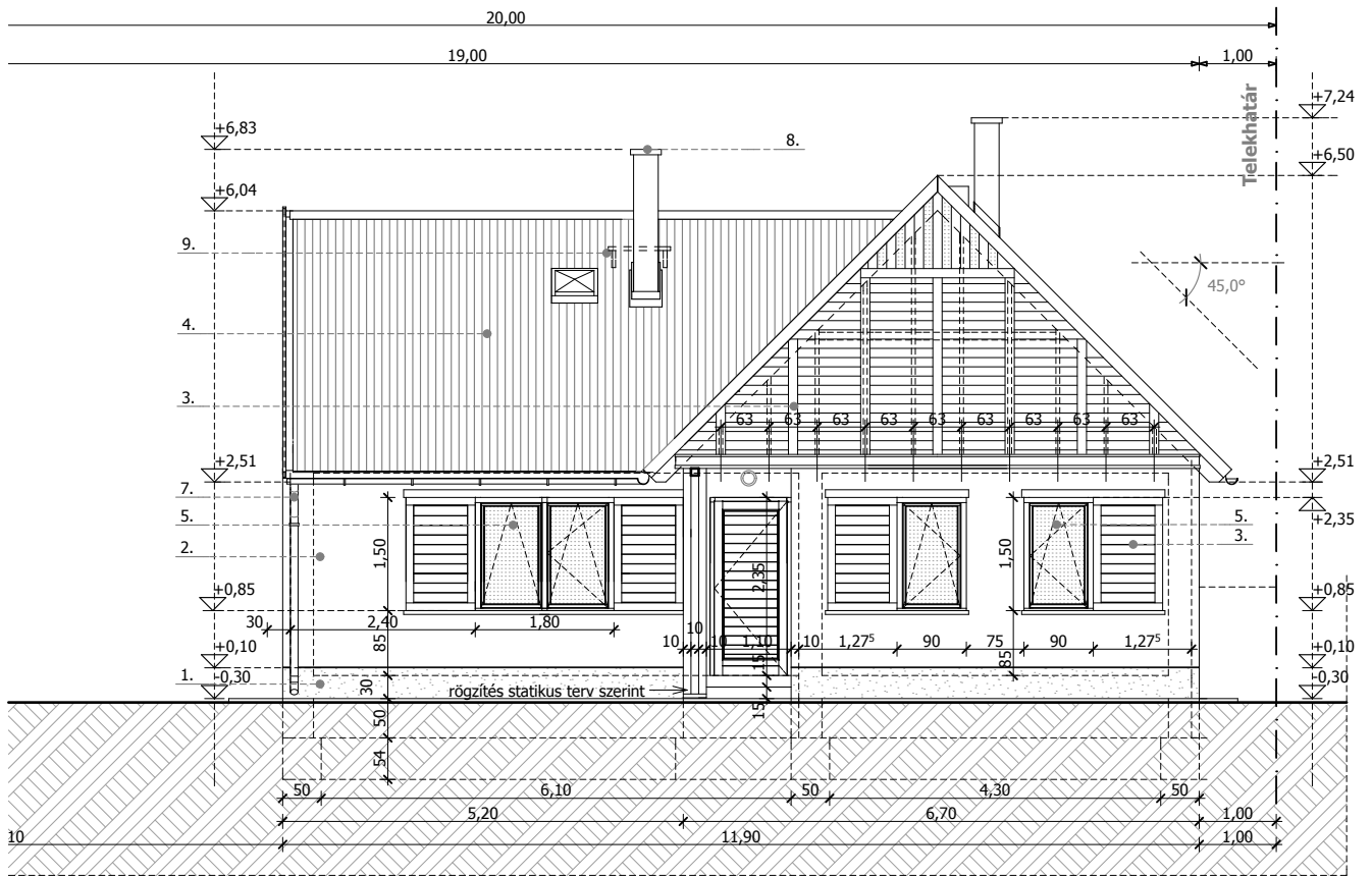
KELETI HOMLOKZAT
